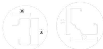
立柱截面图
